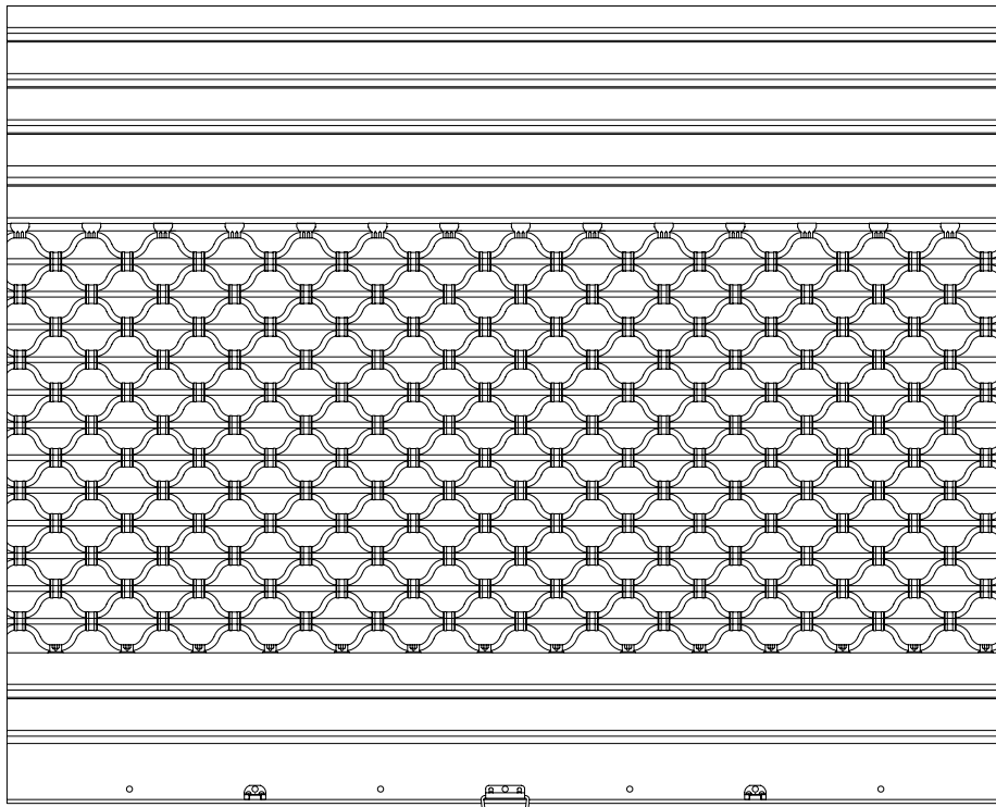
Model T02 ROND 14 VERSTERKTE UITVOERING
