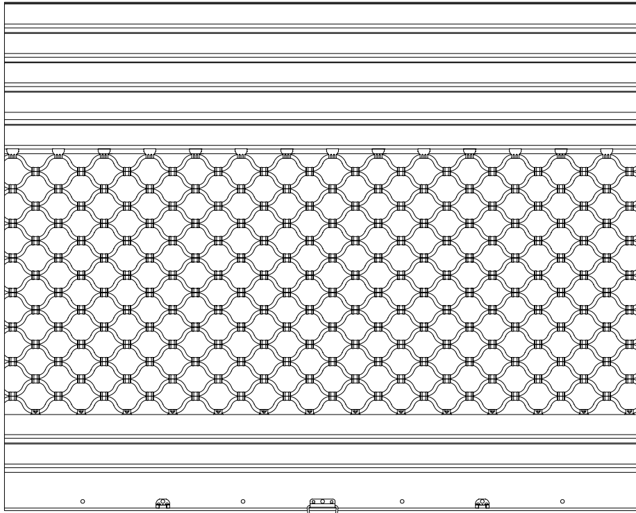
Model FS-T01 ROND 14
